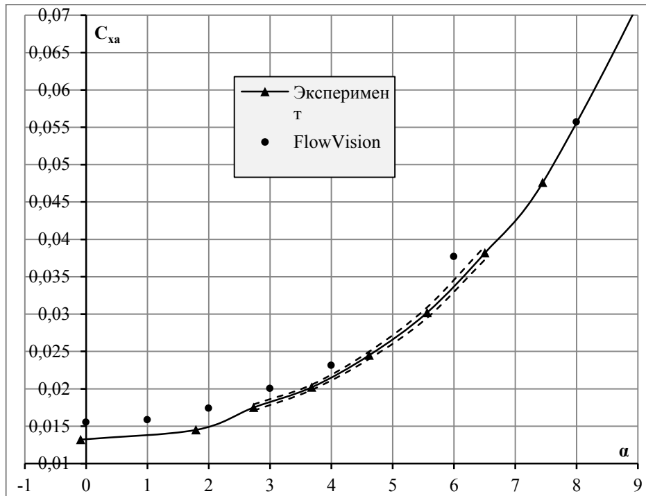
Рис. 5 – График зависимости коэффициента аэродинамического сопротивления от угла атаки
