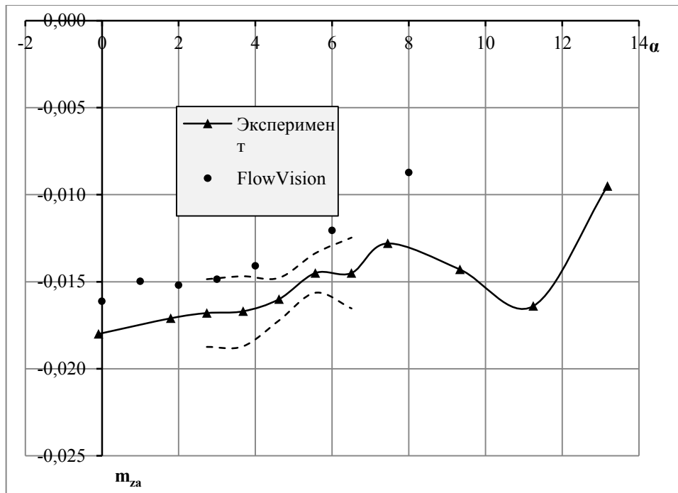
Рис. 6 – График зависимости коэффициента момента тангажа от угла атаки
