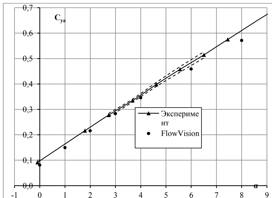
Рис. 4 – График зависимости коэффициента аэродинамической подъемной силы от угла атаки
