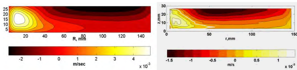
Рис.5. Распределение азимутальной скорости в вертикальном сечении, слева – расчетное поле (осредненное по азимутальной координате), справа экспериментальные измерения (осредненные по времени и азимутальной координате) для P=25 Вт.
