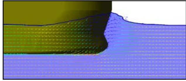
б – носовая оконечность корпуса
