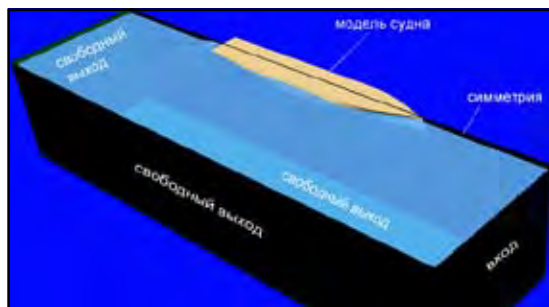
Рис. 2. Расчетная область и граничные условия
