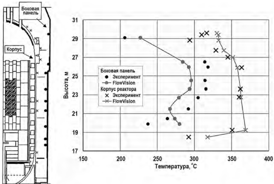
Рис. 4. Распределение температуры на поверхностях корпуса реактора и боковой панели системы охлаждения шахты реактора при работе реактора на мощности 30 МВт
