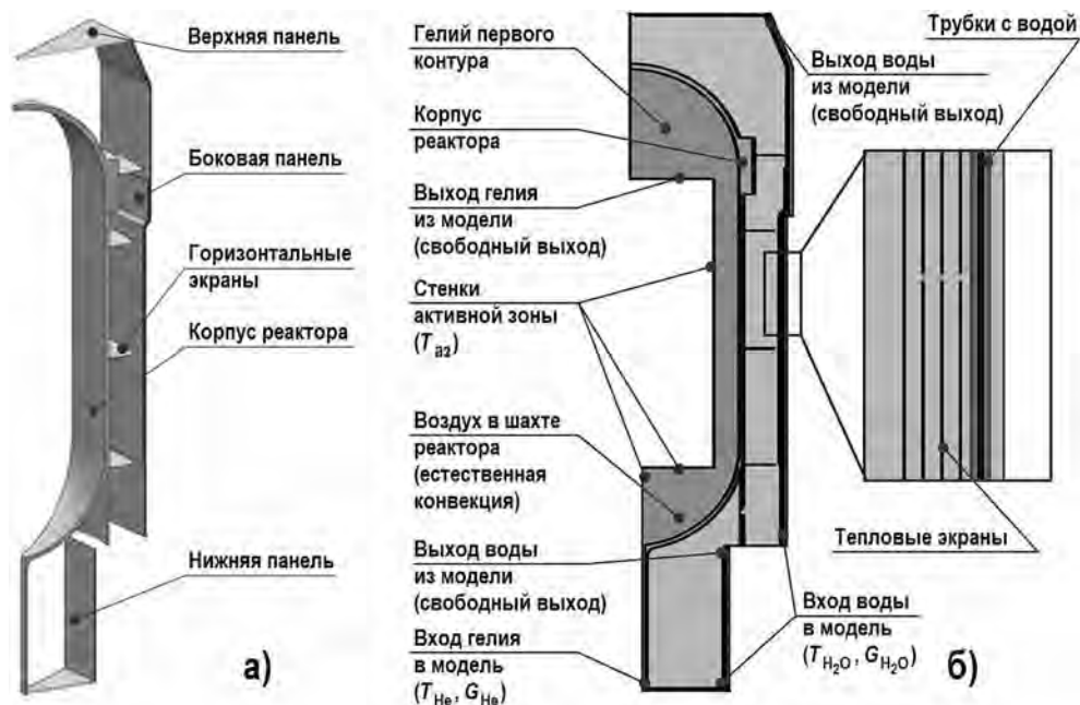
Рис. 3. Геометрическая трёхмерная модель (а) и расчётная модель с граничными условиями в ПК FlowVision (б)
